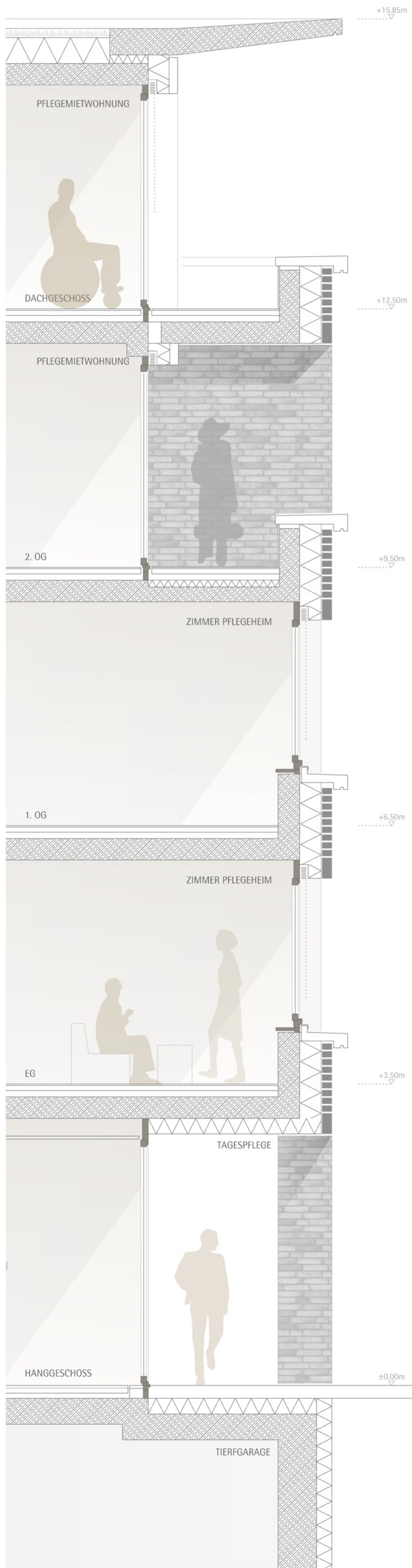
FASSADENSCHNITT_ANSICHT_M 1:20
